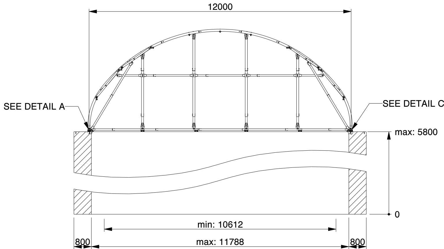
SECTION A-A
