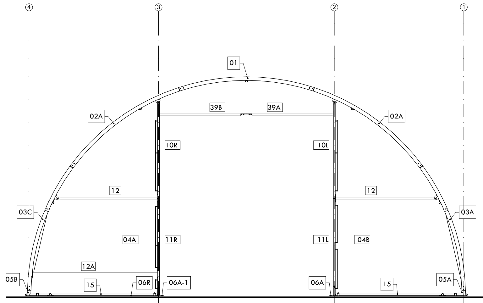
Rückansicht
