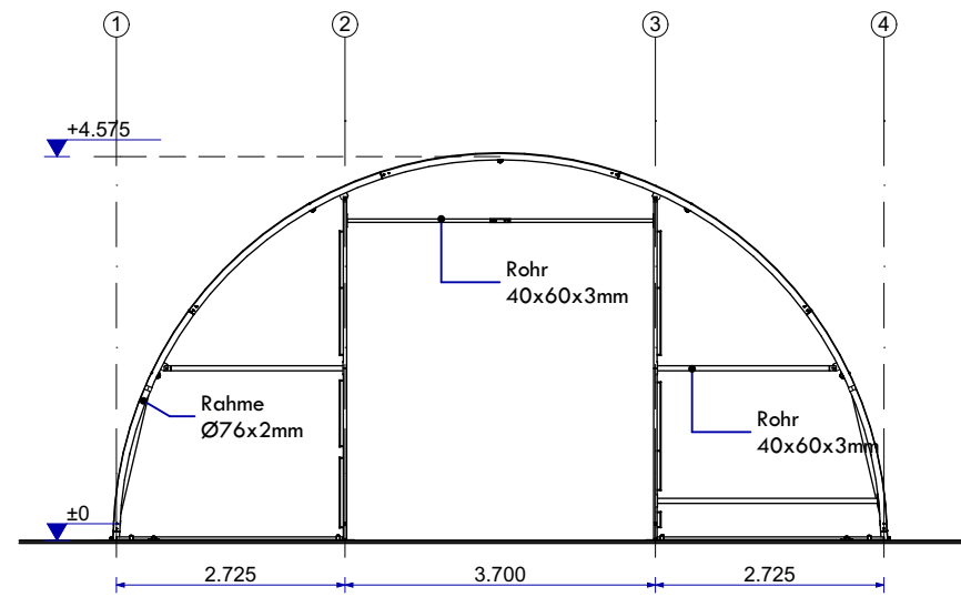
Vorderansicht
