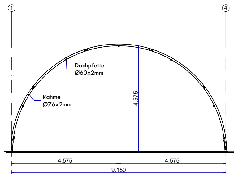
Schnitt A-A
