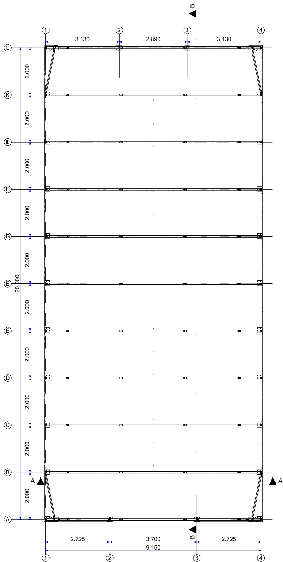
Grundriß
