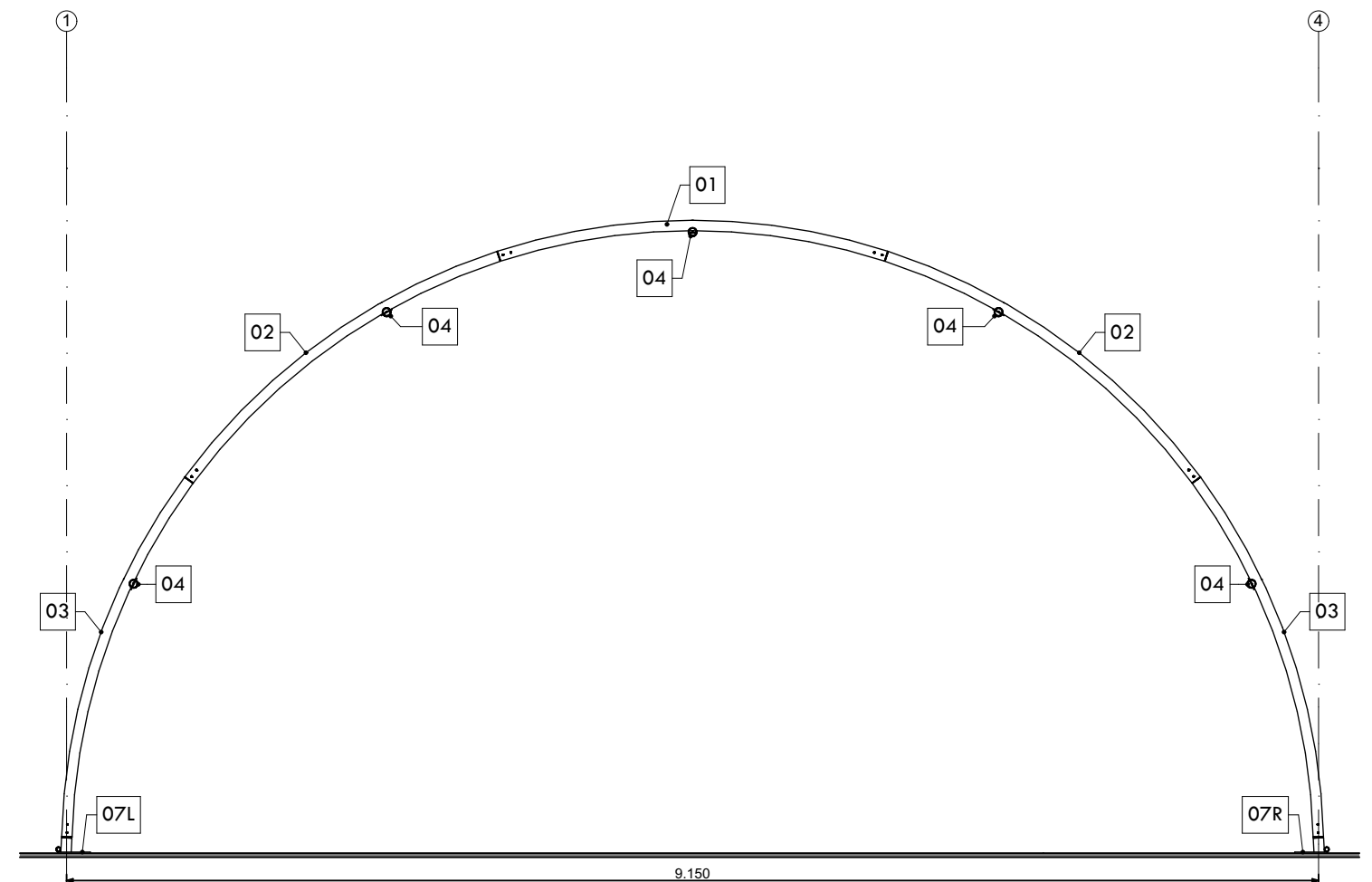
Schnitt
