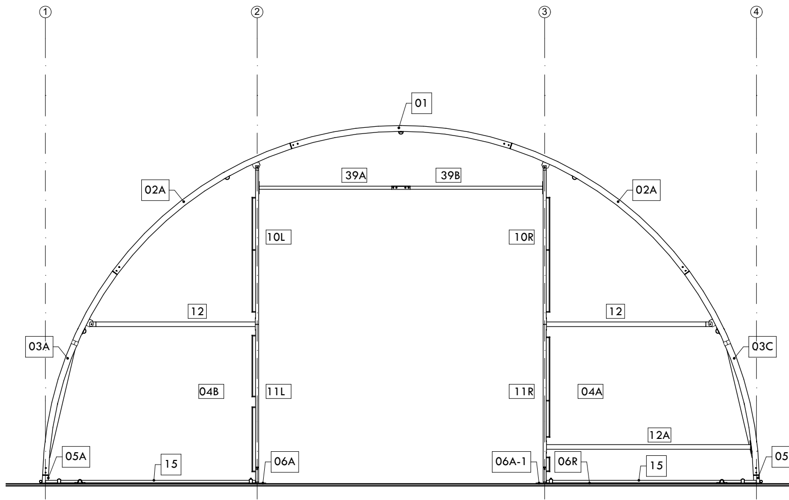
Vorderansicht
