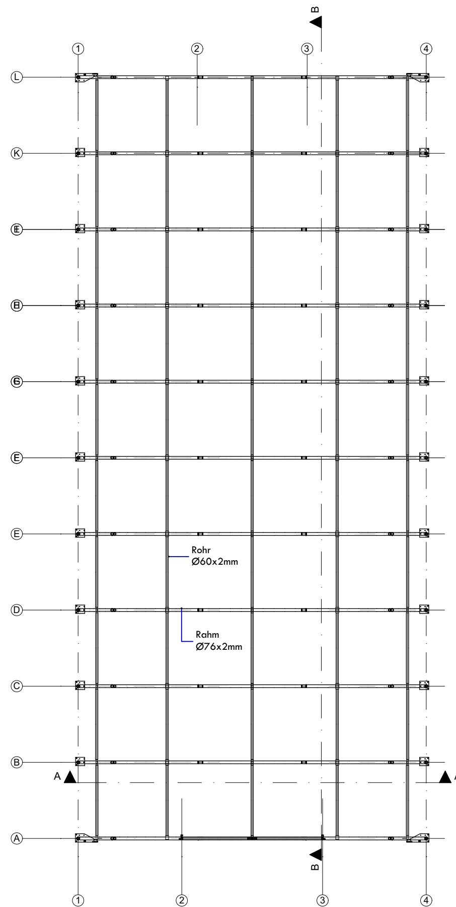
Draufsicht
